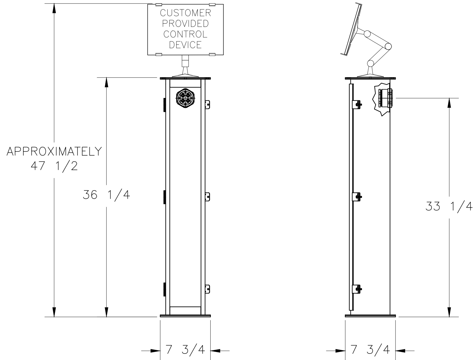
KIOSK1 DIMENSIONS
